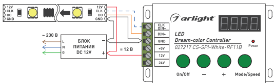
Рис. 1. Подключение контроллера при длине между контроллерами и лентой до 10 м.
