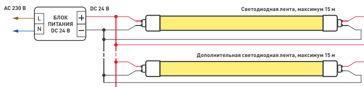
Схема 3. Подключение нескольких светодиодных лент «неон» с двух сторон
