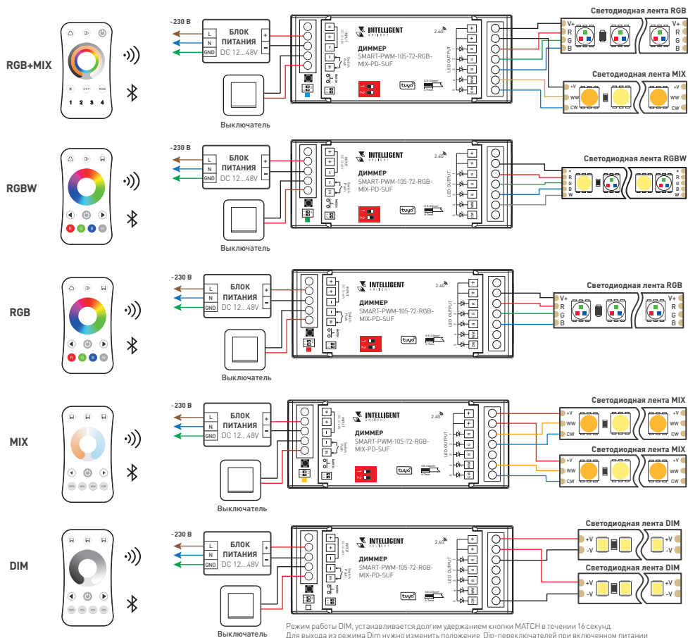
Рис. 1. Схемы подключения диммера SMART-PWM-105-72-RGB-MIX-PD-SUF
