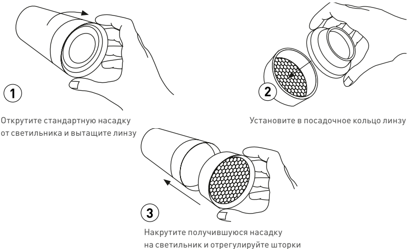
Рис. 2. Установка насадки на светильник
