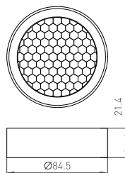
Рис. 1. Чертеж и габаритные размеры
