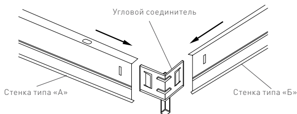
Рис. 1. Сборка углового соединения.
