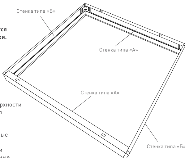
Рис. 1. Сборка углового соединения.
