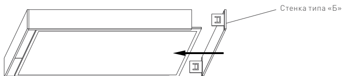
Рис. 3. Установка светильника в рамку.
